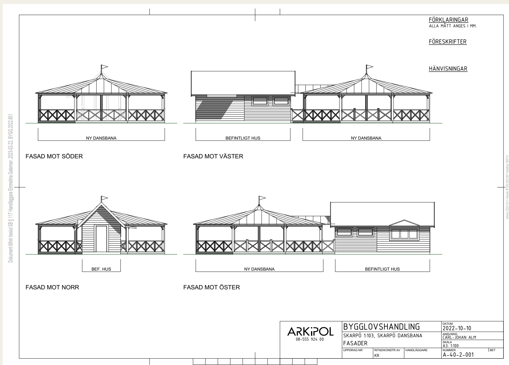
Fasadritningar
